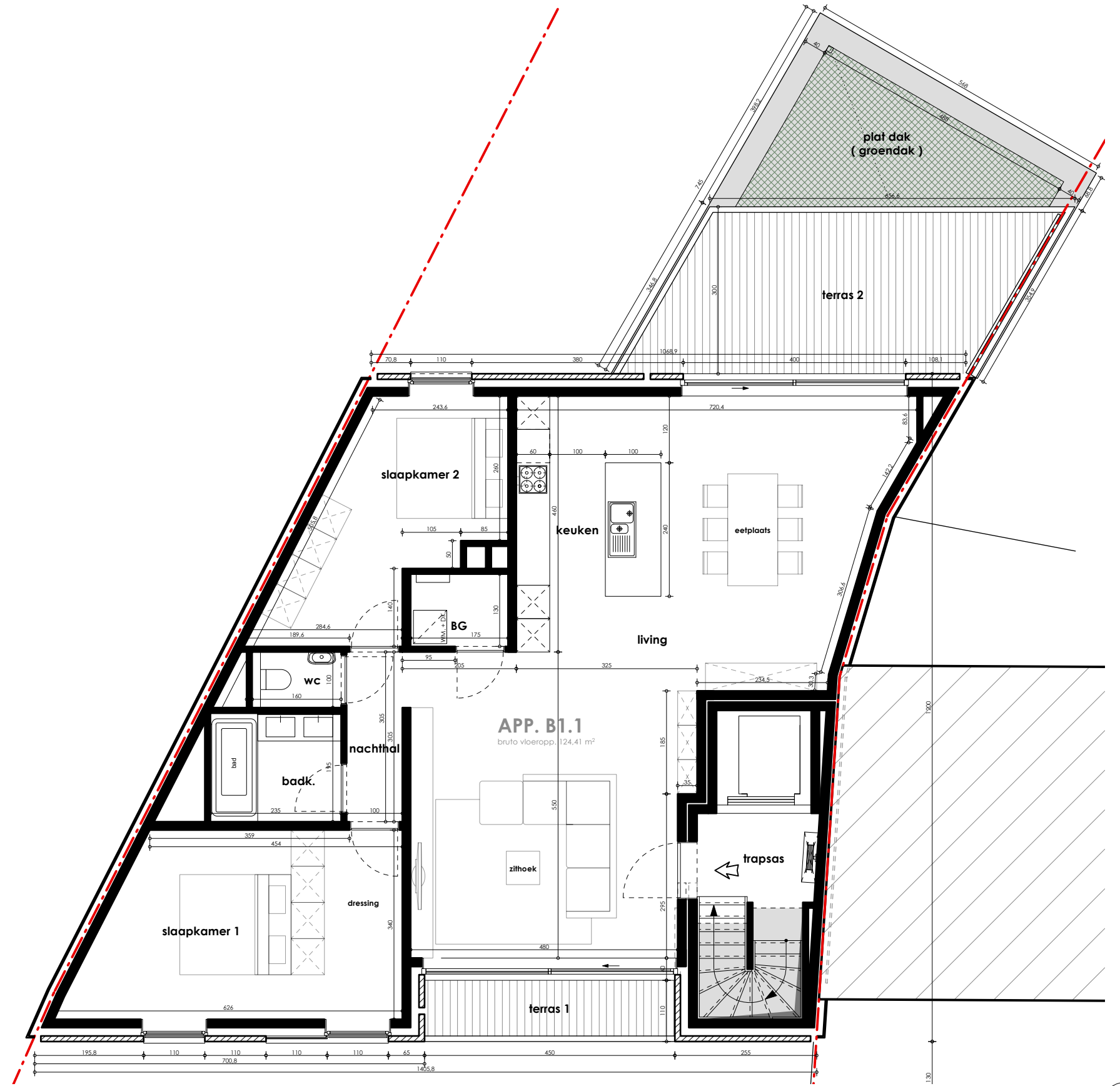
GRONDPLAN
